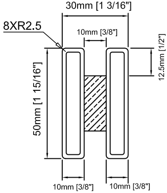
A-A Detail
