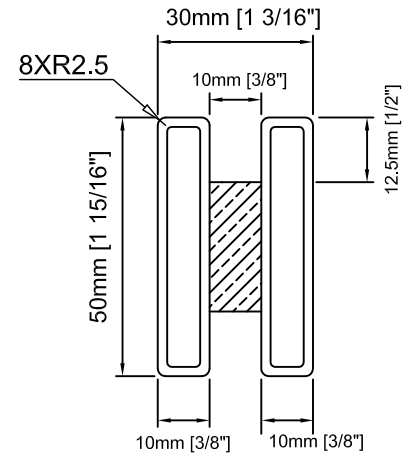
A-A Detail
